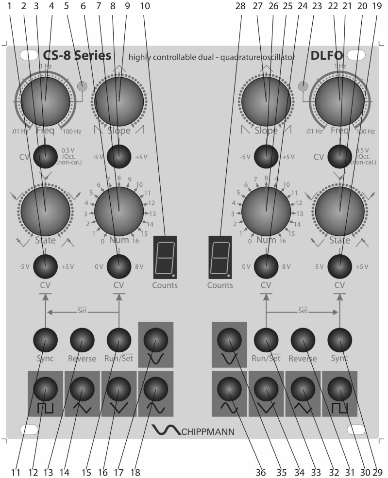
Abb. 1 DLFO Frontseite
